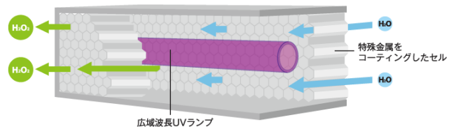
NCCセルの構造
